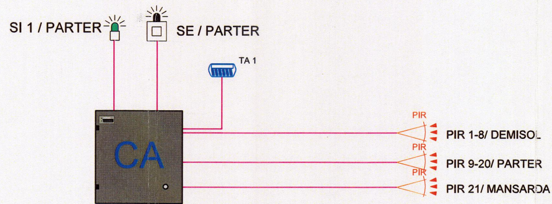
Schema bloc sistem antiefracție
