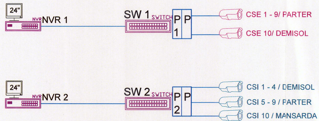
Schema bloc sistem supraveghere video
